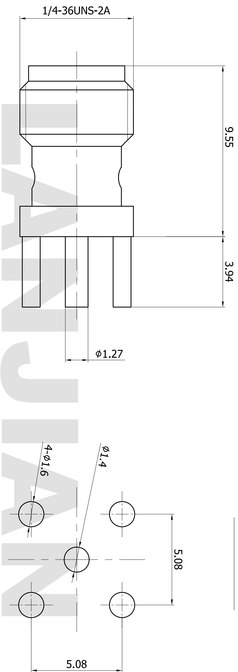
安装孔尺寸
