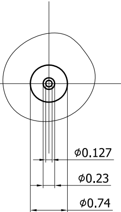
A部局部视图(20:1)
